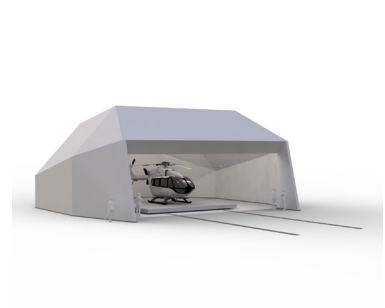
V 02 L 16,4 | W 15,5 | H 7,2
